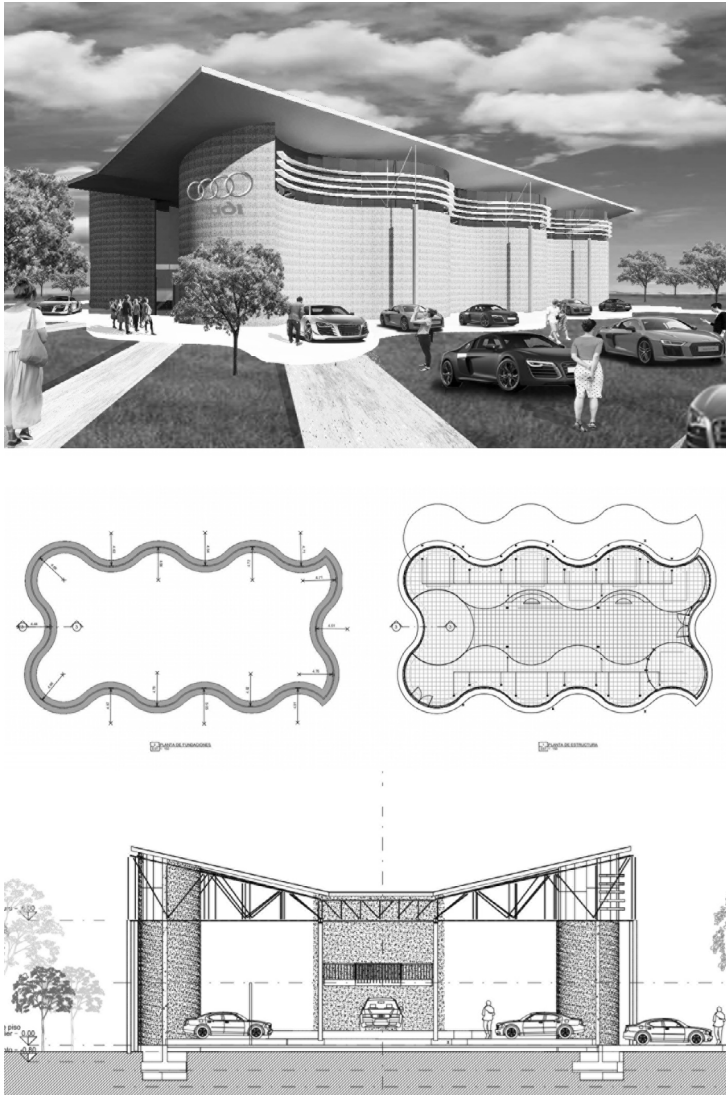
Figura 3. Modelo BIM de construcción impresa-3D (fuente: García-Alvarado et al. 2020).
